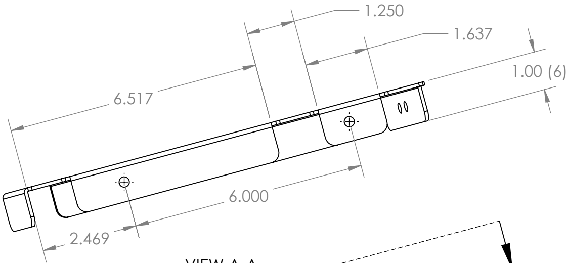
VIEW A-A
